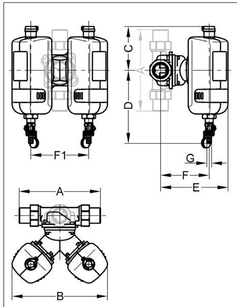
Abb. 10: Einbaumaße JMFI 1 1/2"
